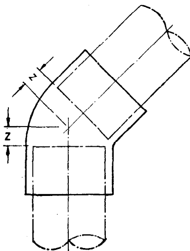
FIG. 1 45° Elbow
